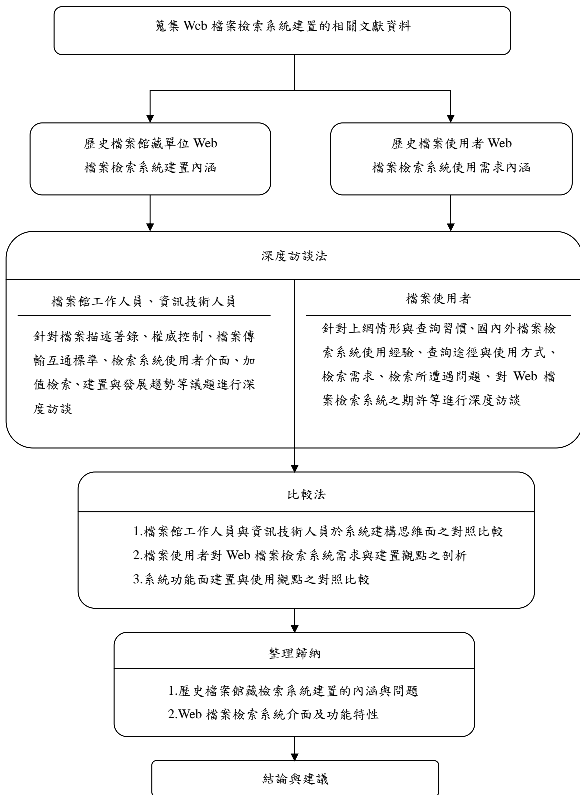
圖 3.1 研究架構圖
