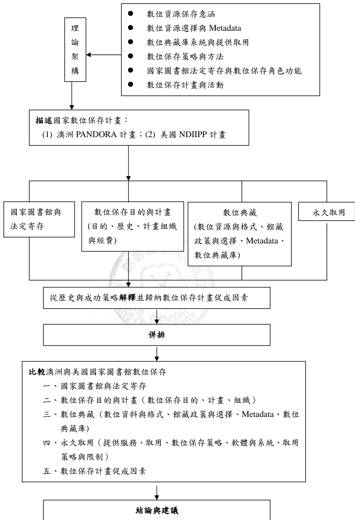
圖 3-1 研究架構圖
