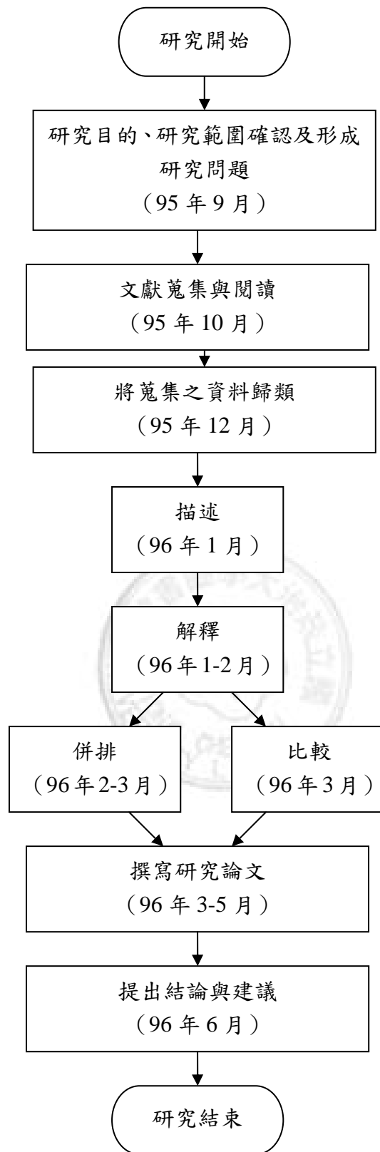
圖 3-2 研究流程圖
